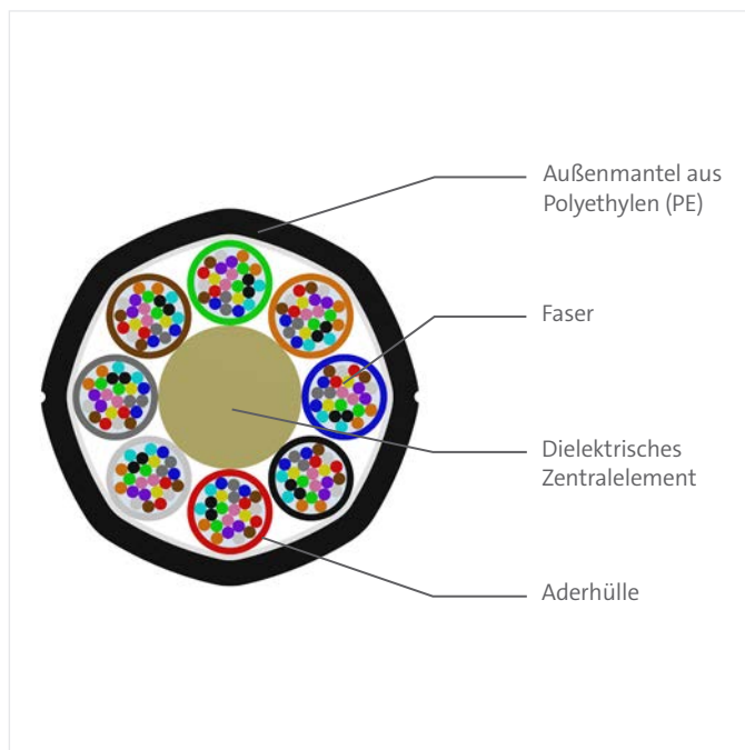
Kabelquerschnitt der Katalognummer: 192ZH4-Y3C42ADE
